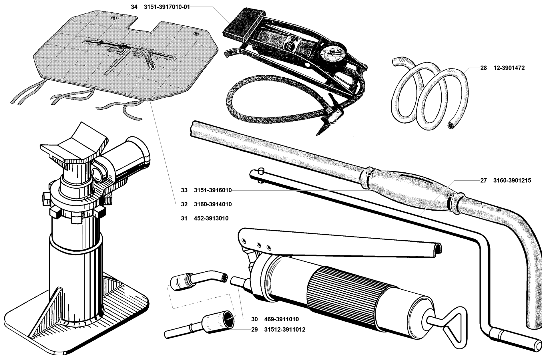
Рис. 106. Инструмент водителя и принадлежности (3901)/2, шприц для смазки (3911), домкрат (3913), утеплители (3914), насос топливopеpекачивающий (3916), насос для накачивания шин (3917)
